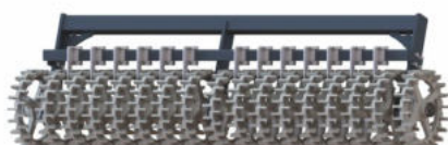
Wał crosskill Ø500 mm
